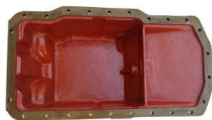
E2NN6676A Carter de motor - Ford 5000, 6600
